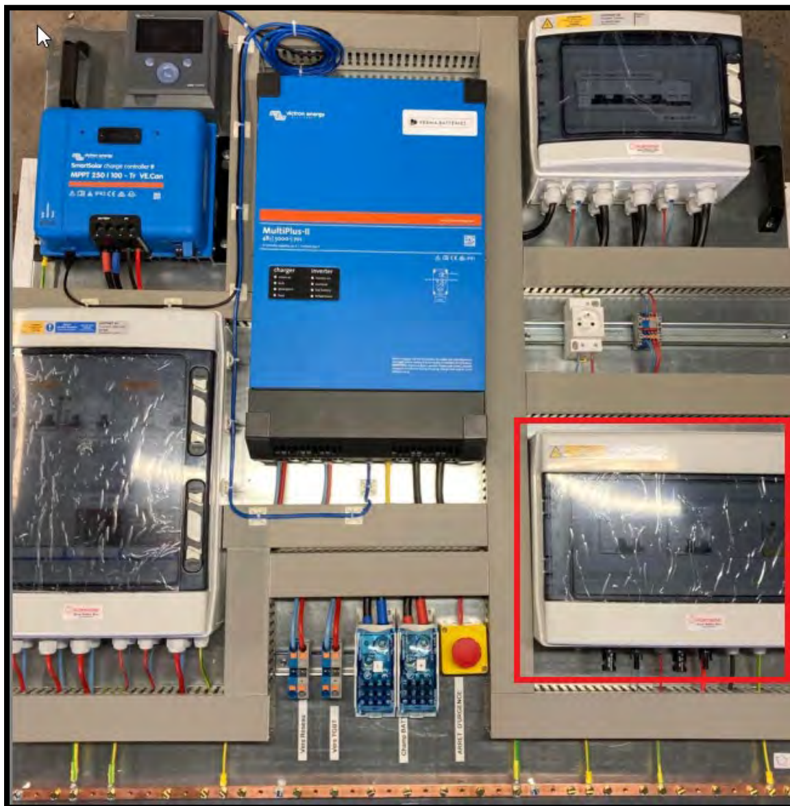
Emplacement du coffret « solaire » sur la platine
