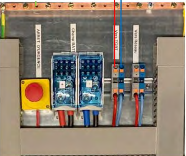
Vers bornier ressort « Vers TGBT »
