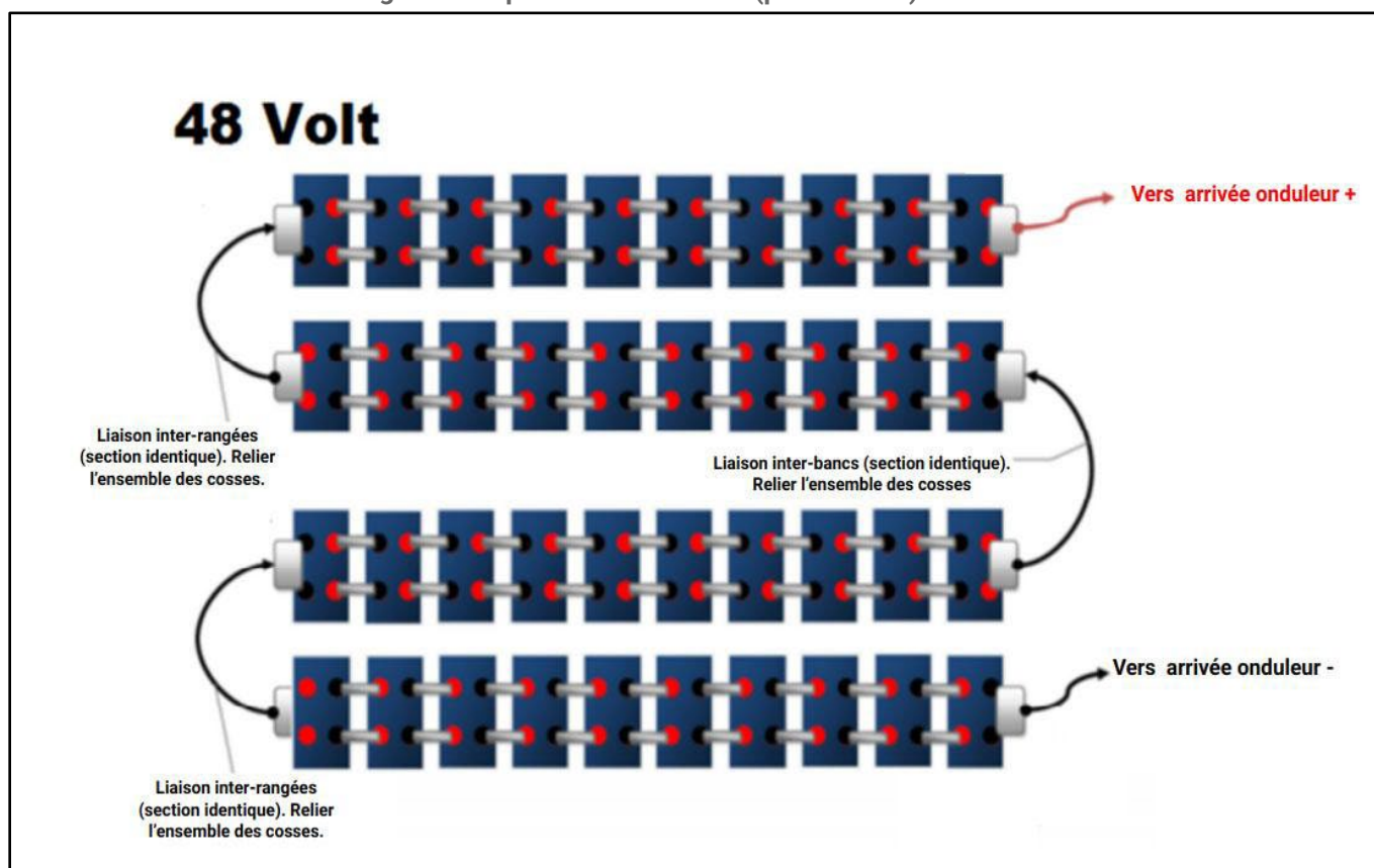
Fig. 7. Exemple de mise en série (parc en 48V)
