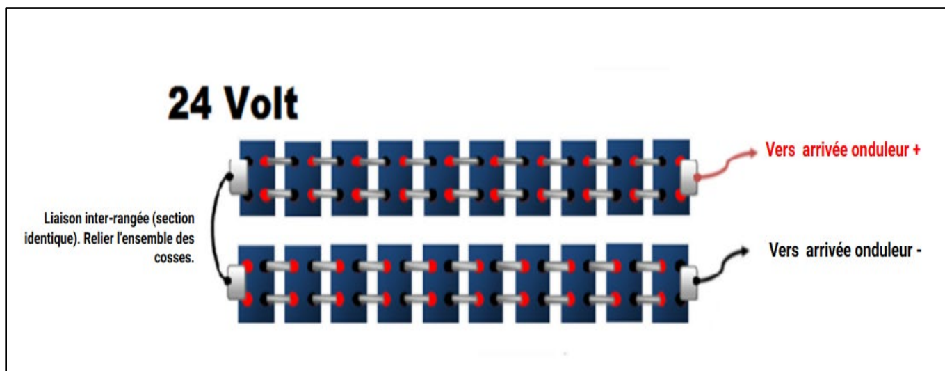
Fig. 6. Exemple de mise en série (parc en 24V)
