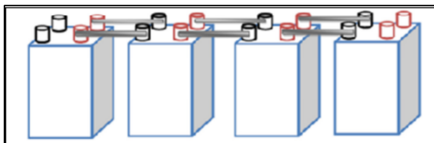
Fig. 8. Vue de profil (branchements inter-cellules).
